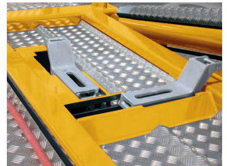
Butées de bennes escamotables / réglables sur structure avec protections abaissées
